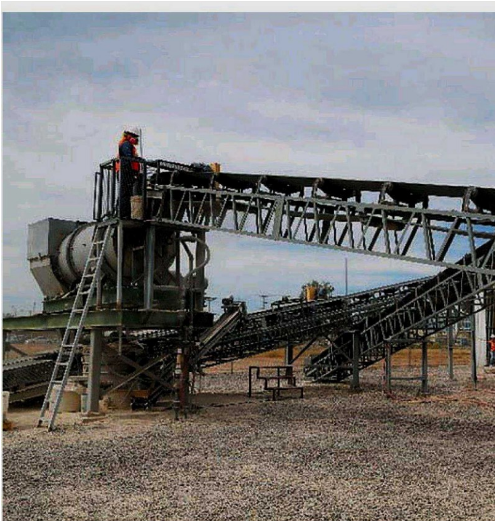
La planta piloto de litio de Bacanora, Sonora, que forma parte de Sonora Lithium Project, desarrollado por las empresas Bacanora Lithium y Gangfeng Lithium /CORTESÍA BACANORA LITHIUM
